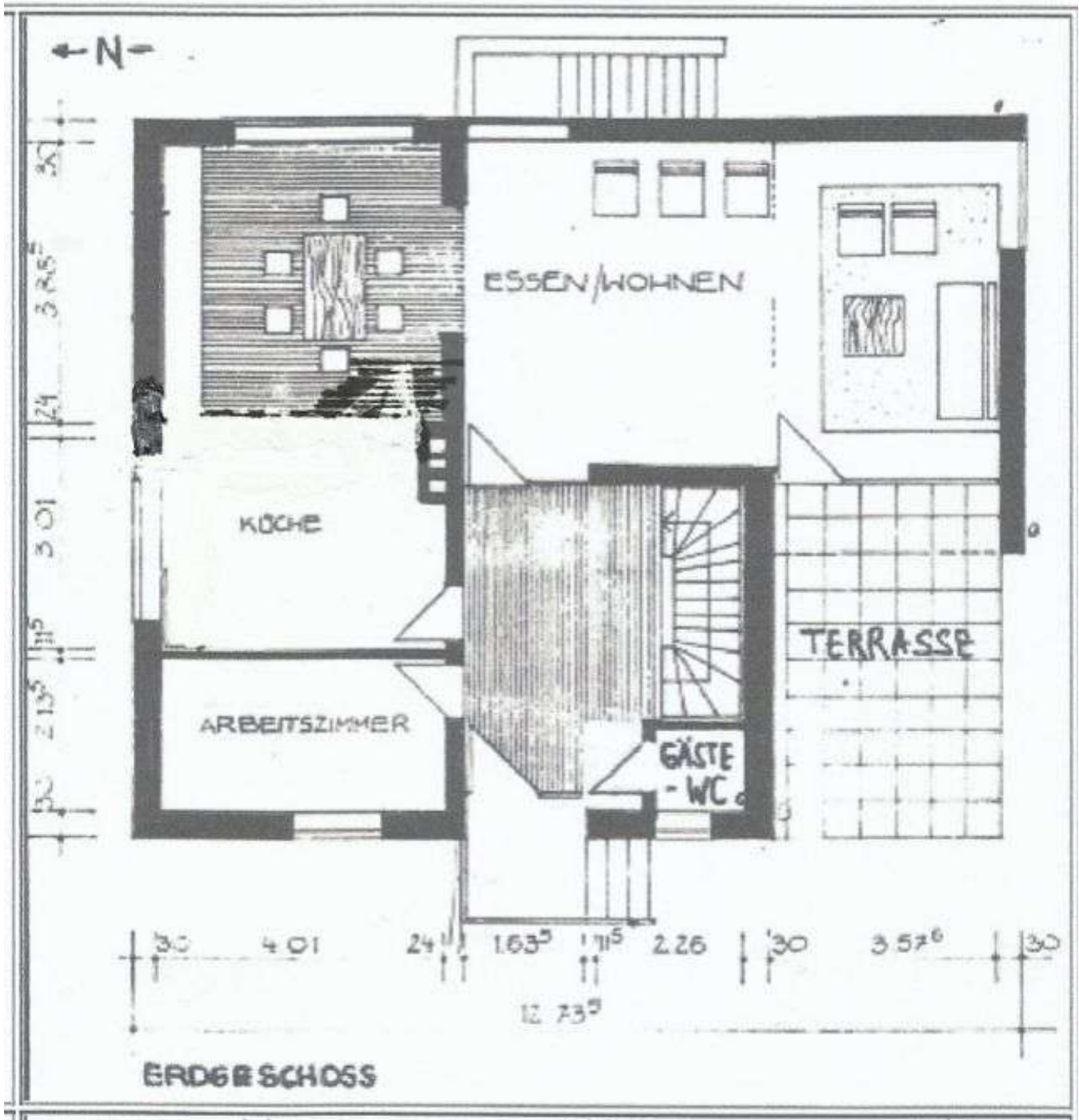
EG Grundriss
