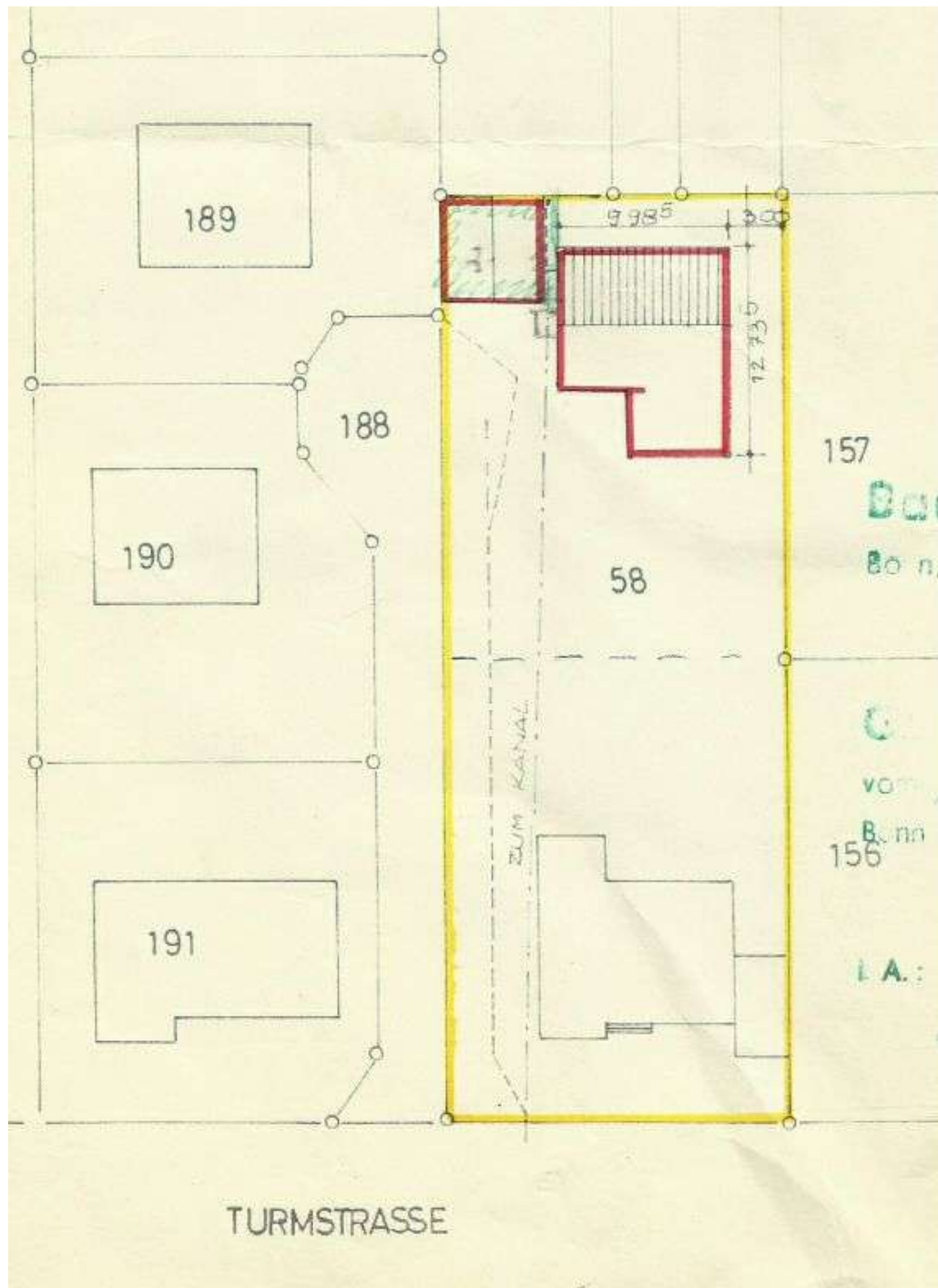
RT24Lageplan
