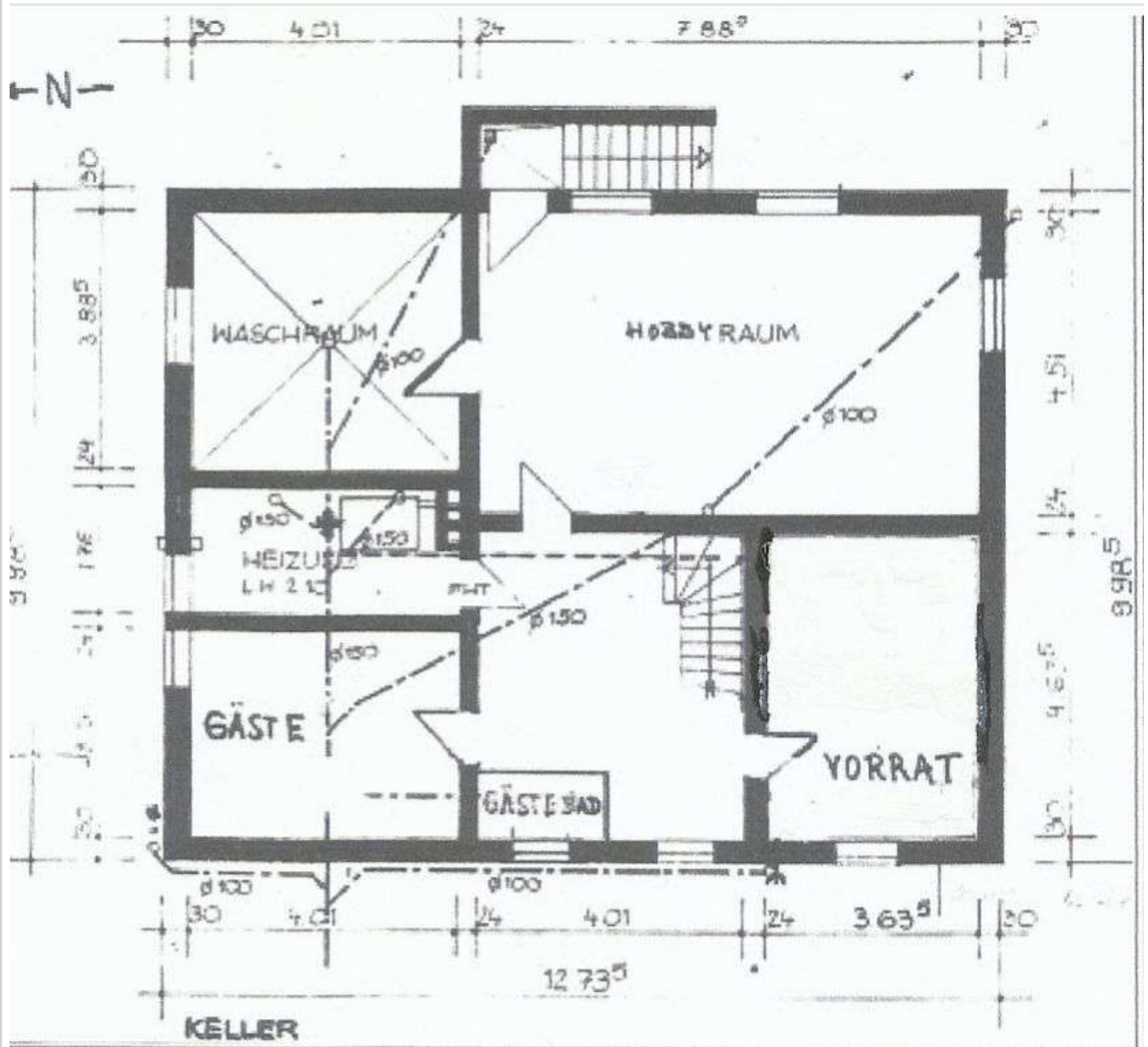
UG Grundriss
